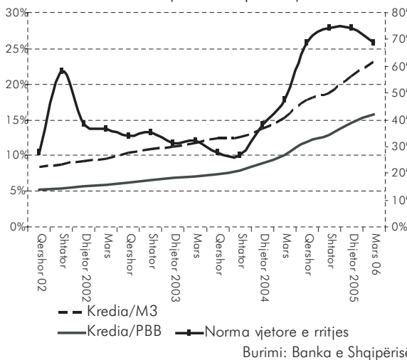
Grafik 12. Raporti i kredisë ndaj PBB-së dhe M3 (shkalla majtas) dhe norma vjetore e rritjes së kredisë (shkalla djathtas).
